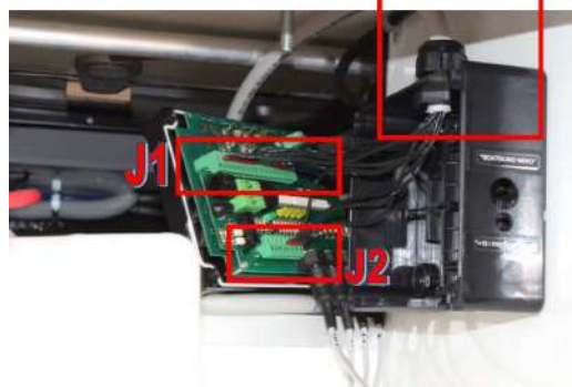
Câbles de connexion avec la pompe hydraulique
